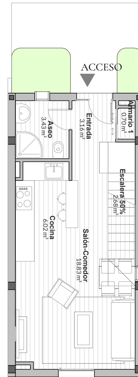
PLANTA BAJA
