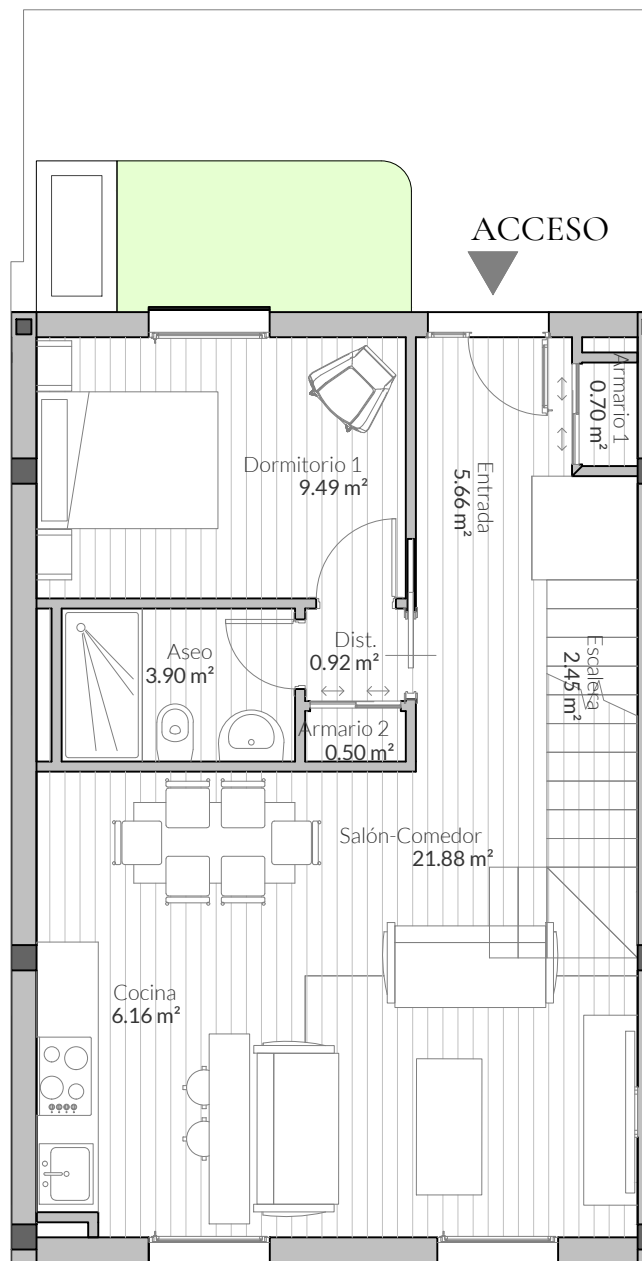
PLANTA BAJA
